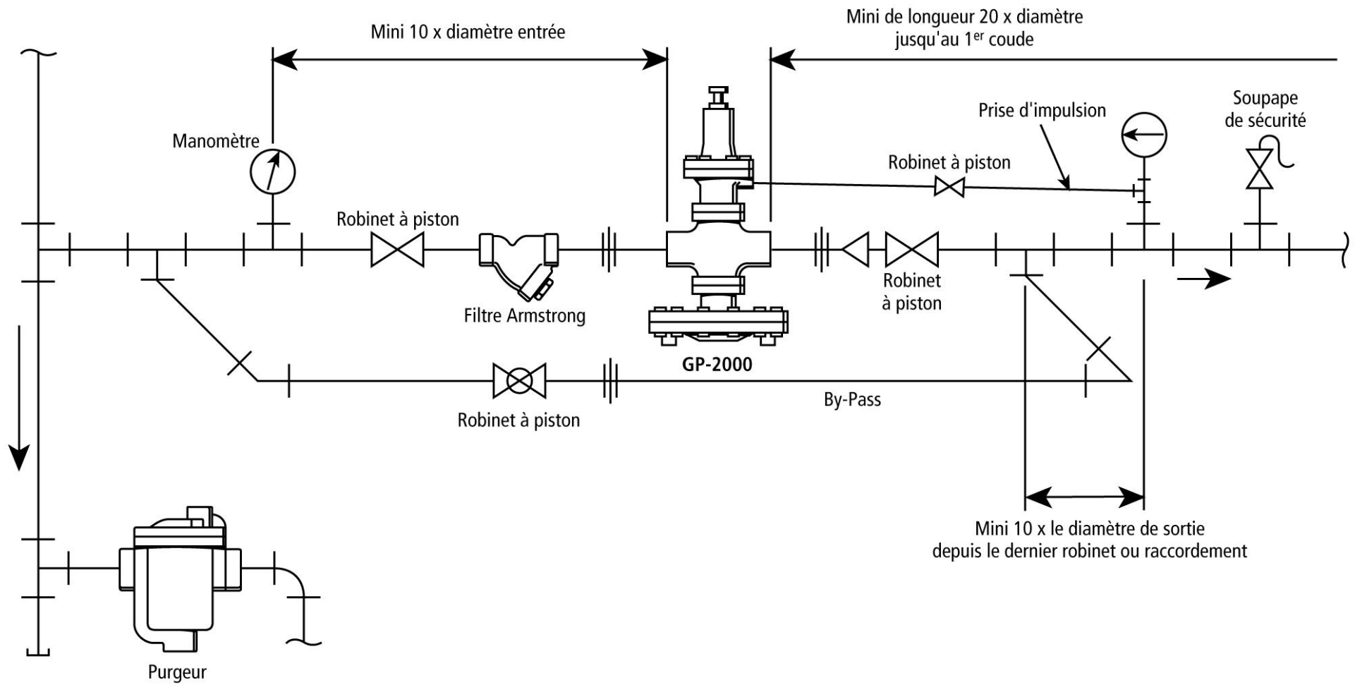
Schéma de principe du détendeur piloté
